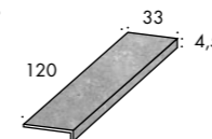
gradone - step *33-120-4,5 cm *13" . 47" . 1 7/8"
