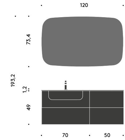
Teso — 02 L 120,6 × P 37,5/43 cm
