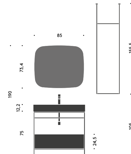
Teso — 10 L 88,8 × P 50,5 cm
