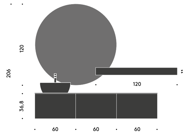
Teso — 03 L 180,6 × P 50,5 cm (L 210 con sporgenza mensola)
