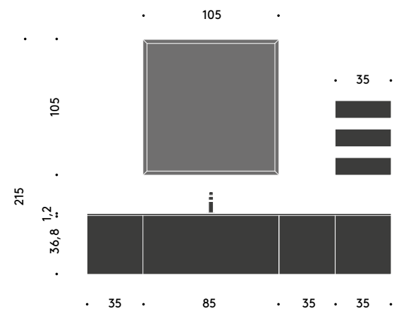
Teso — 06 L 190,6 × P 50,5 cm
