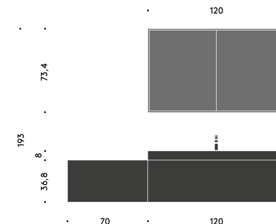
Teso — 12 L 190,3 × P 50,5 cm
