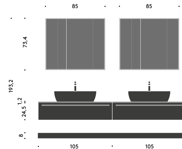
Teso — 09 L 210,6 × P 50,5 cm
