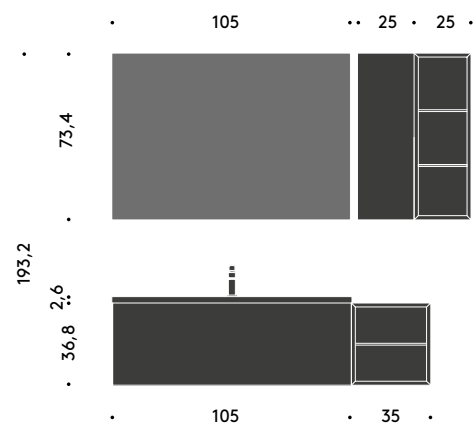
Teso — 05 L 140,3 × P 50,5 cm (L 158 con sporgenza pensile)
