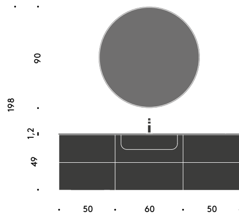
Teso — 07 L 160,6 × P 37,5/43 cm
